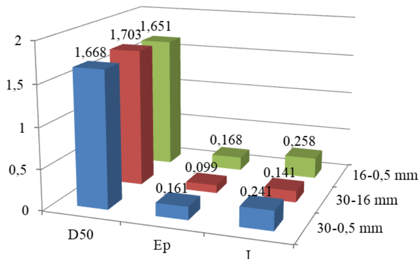
Rys. 2. Wpływ uziarnienia nadawy na parametry rozdziału klasy ziarnowej 30-0,5 mm – Rozdział II [4]
