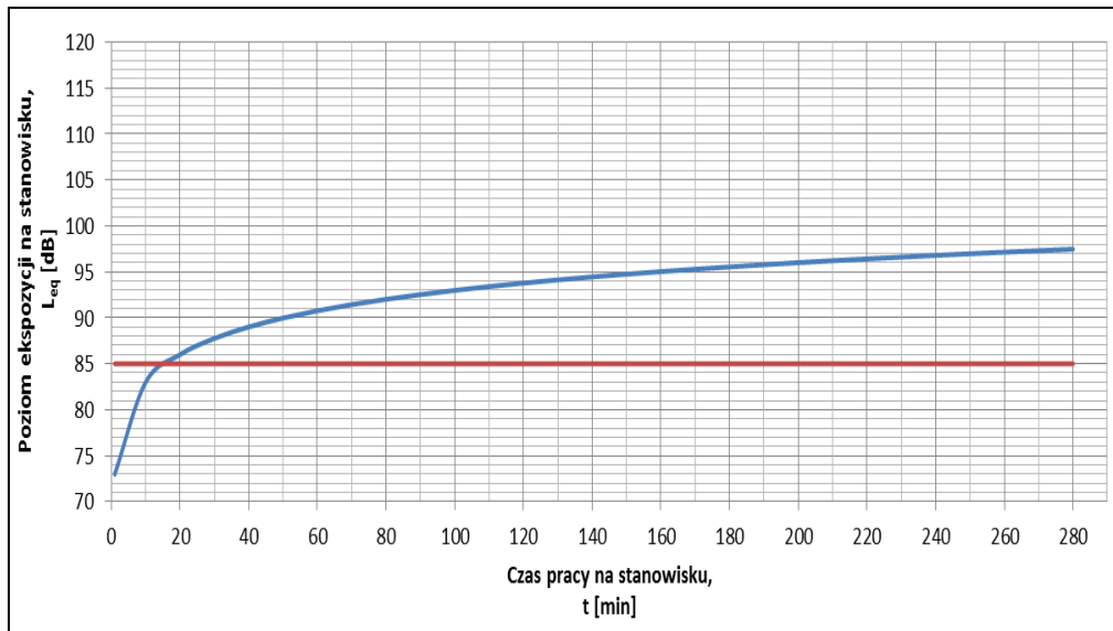
Rys. 1. Poziom ekspozycji na stanowisku obsługi młynów kulowych i rekuperacji - czas pracy dla dziennego poziomu ekspozycji L_{EX,sh} = 85,0 dB; t = 17 min [2]
